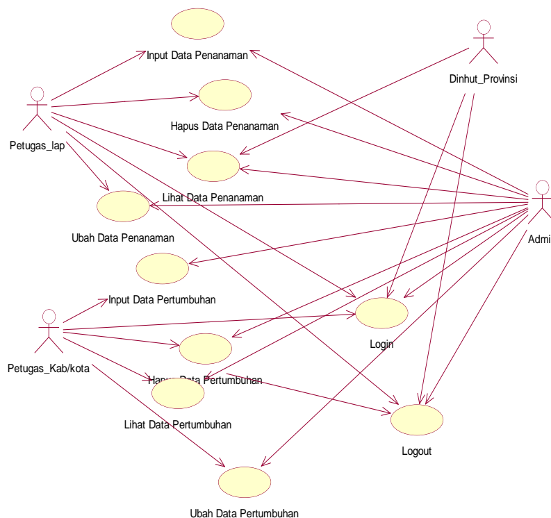
Gambar 3. Use Case Diagram Sistem Pemantau Penanaman Pohon
