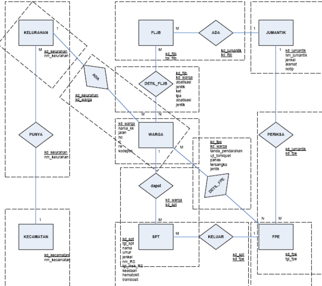
Gambar 6: Transformasi ERD ke bentuk LRS
