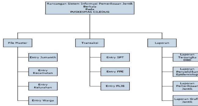
Gambar 8: Stuktur Tampilan
