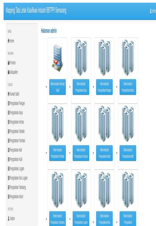
Gambar 12. Implementasi Menu Utama
