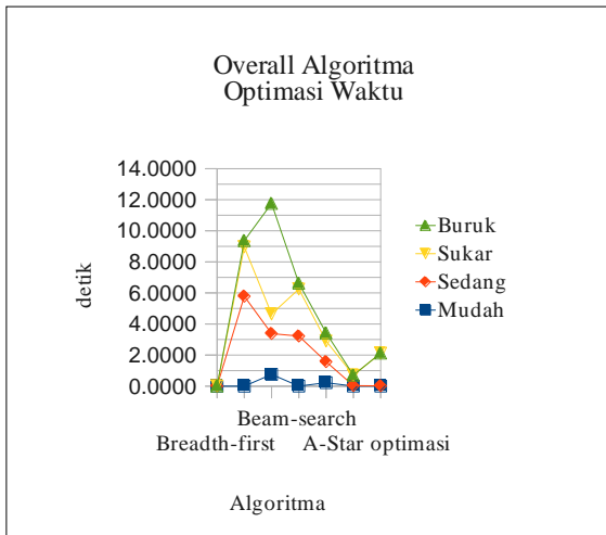
Grafik 1. Overall Algorithma pada optimasi waktu
