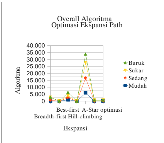
Grafik 2. Overall Algorithma pada ekspansi path
