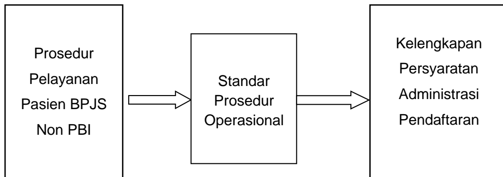
Gambar 3.1 Kerangka Konsep
