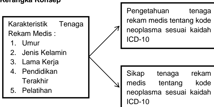
Gambar 3.1 : Kerangka Konsep
